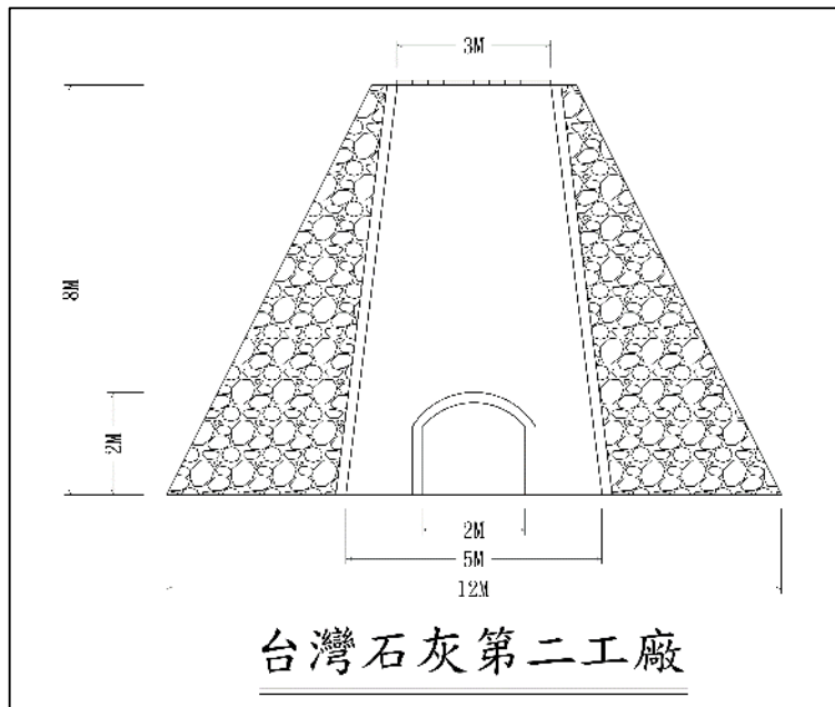
圖 49 臺灣石灰第二工場石灰窯剖面圖
