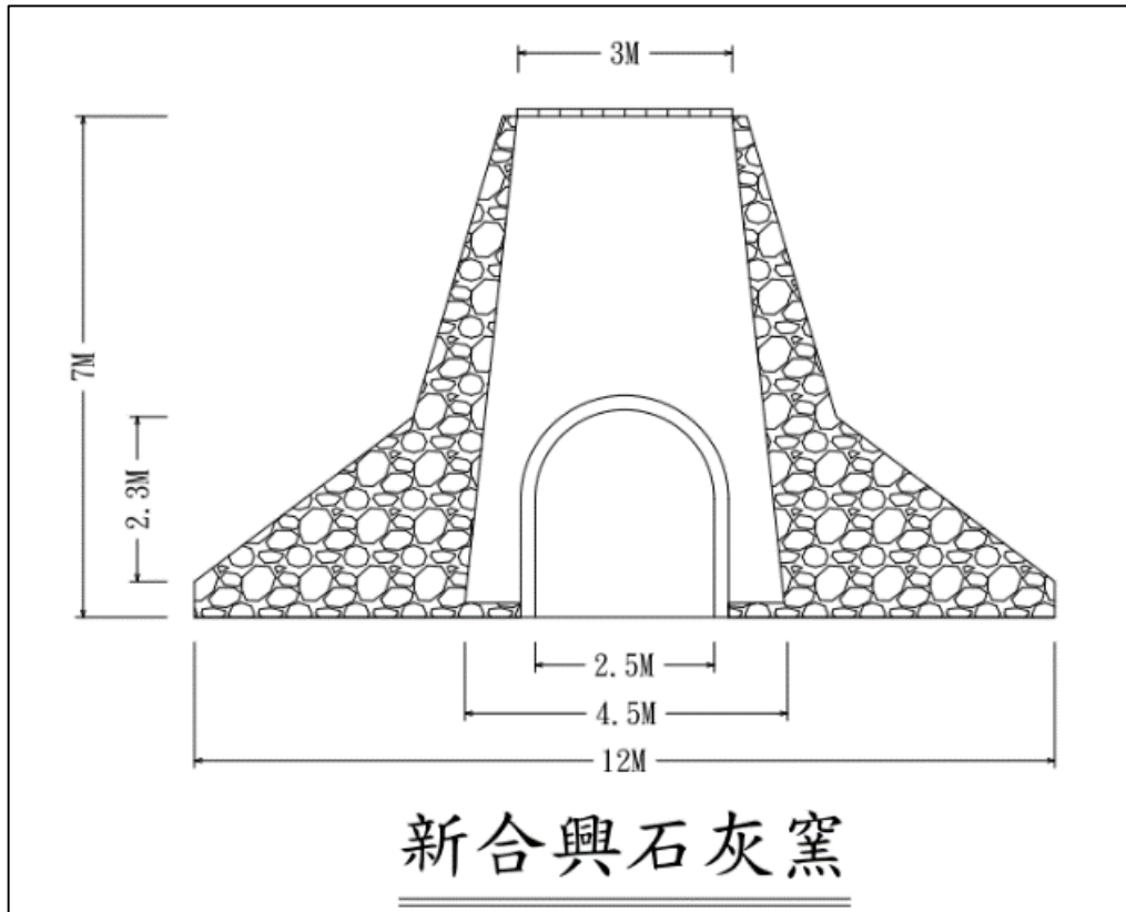
圖 79 新合興石灰窯剖面圖
