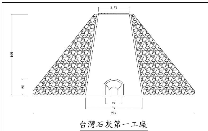
圖 46 臺灣石灰工場石灰窯剖面圖
