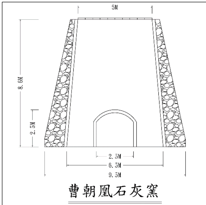
圖 33 曹朝鳳石灰窯剖面圖
