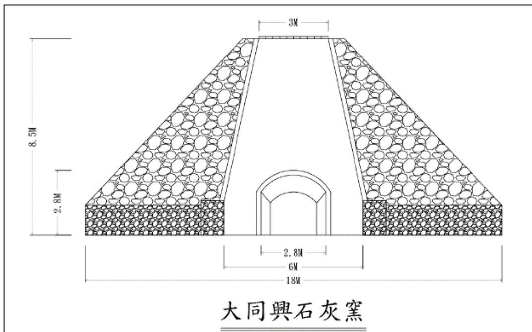
圖 65 大同興石灰窯剖面圖
